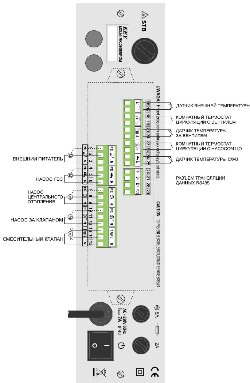
Схема подключения регулятора RK-2006SPGM+MZLN.
