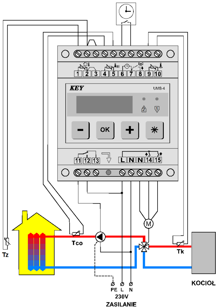
Rysunek 3. Schemat podłączenia modułu UMS-4PR.
